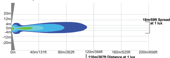
DURA-410 | 9891132 - 10° Beam
