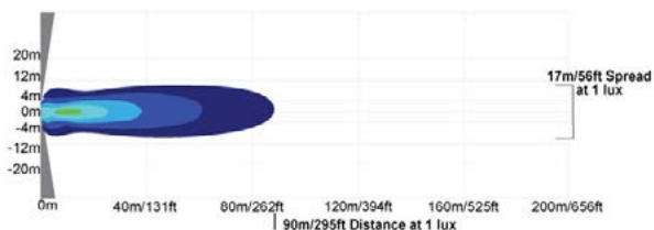
DURA-M4M | 9911649 - 10/25° Beam
