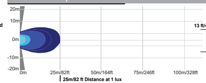
XIL-MX160 | 9113807 - 60° BEAM
